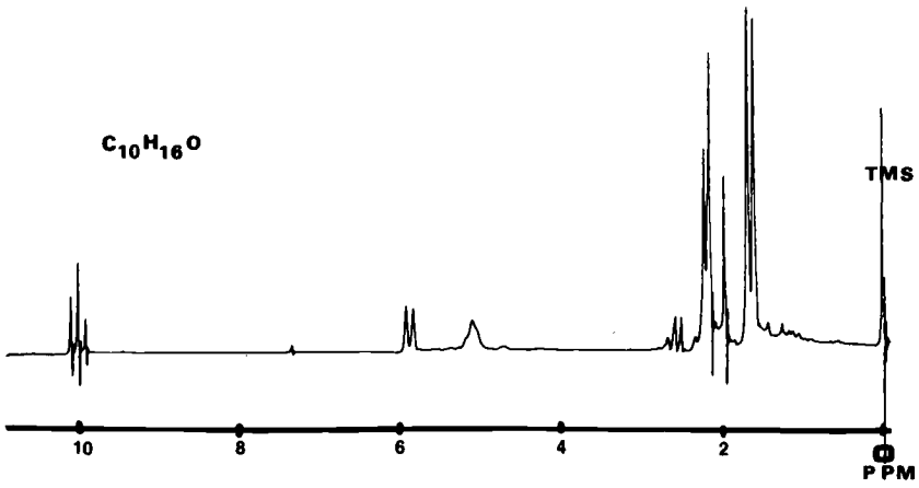
FIG. 5—NMR spectrum of citral.
