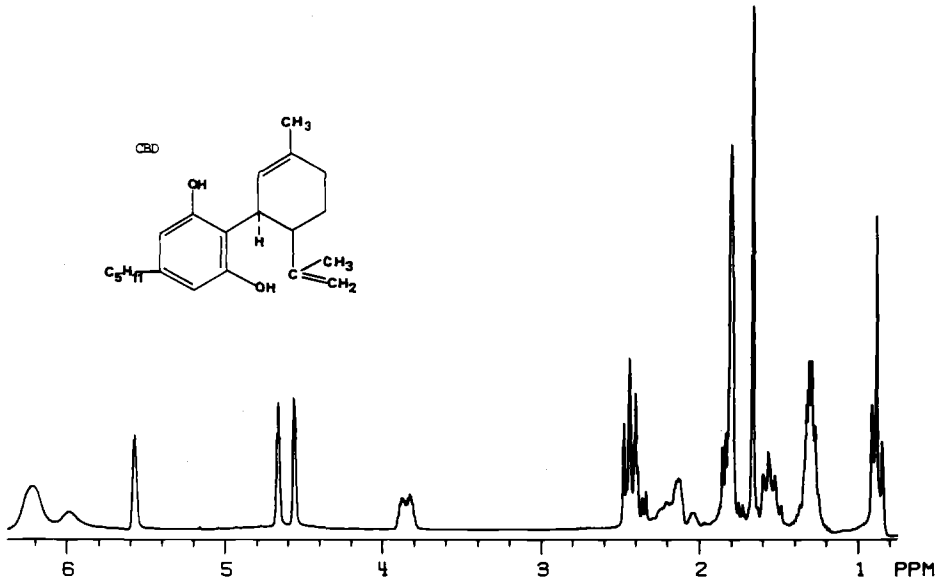
FIG. 12—NMR spectrum of cannabidiol.
